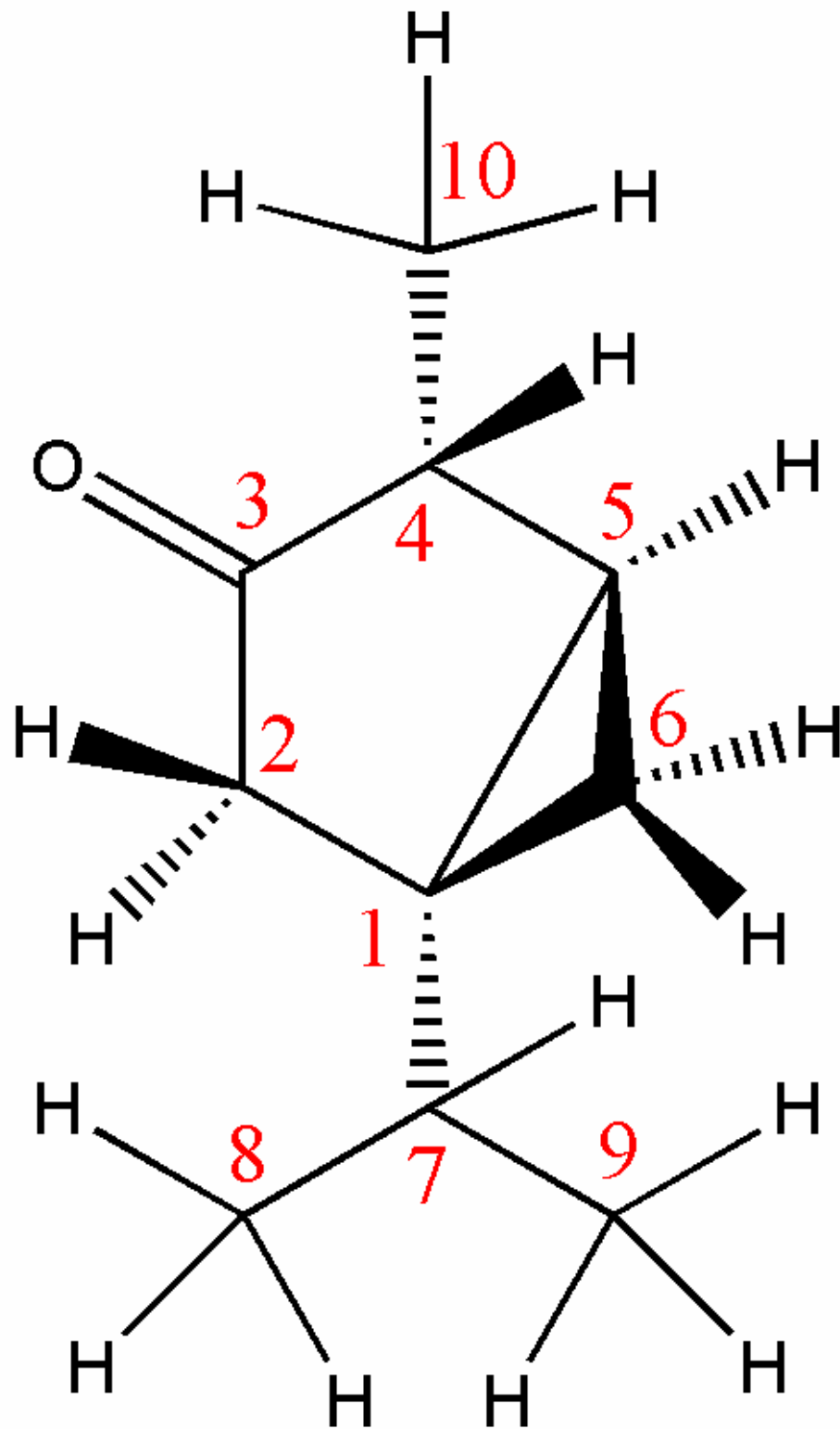
Abb. C-1 \alpha -Thujon
