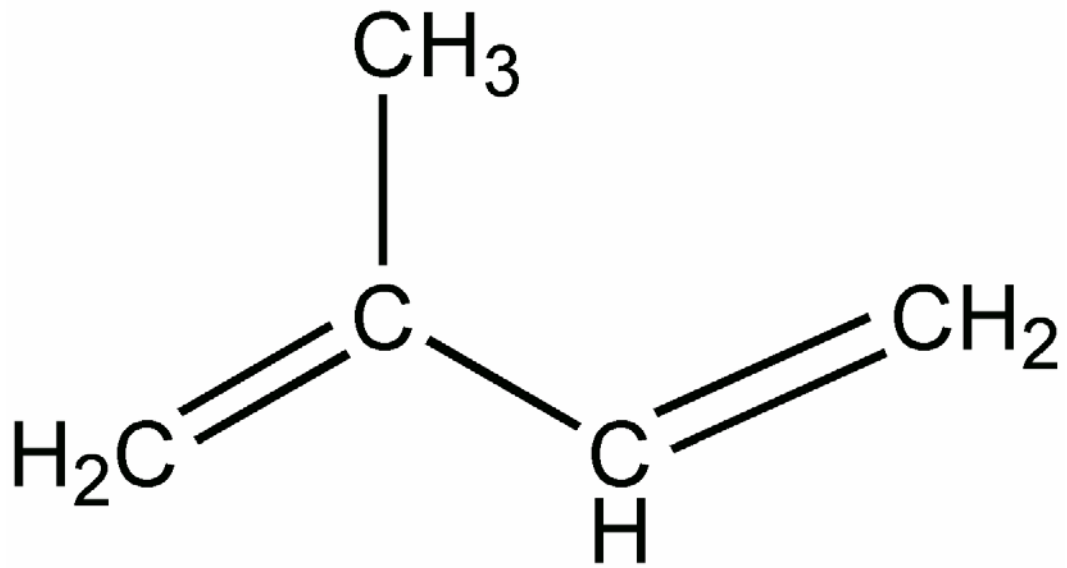
Abb. C-4 Isopren, 2-Methyl-buta-1,3-dien oder Isopentilen
