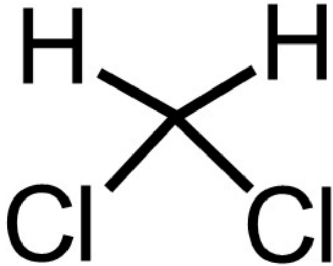
Abb. C-6 Dichlormethan, Methylenchlorid
