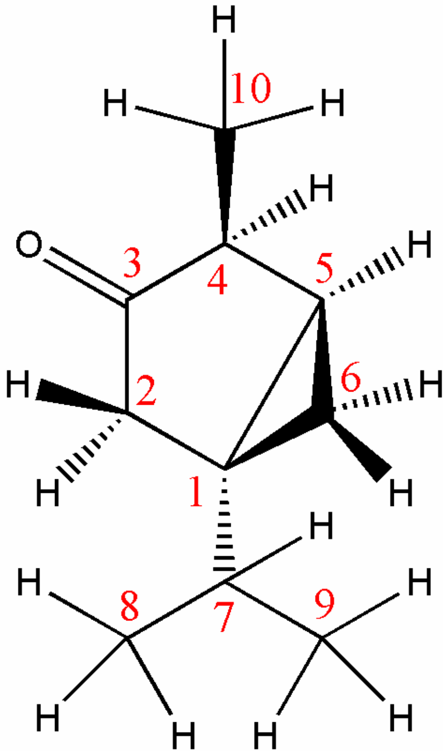
Abb. C-2 \beta -Thujon
